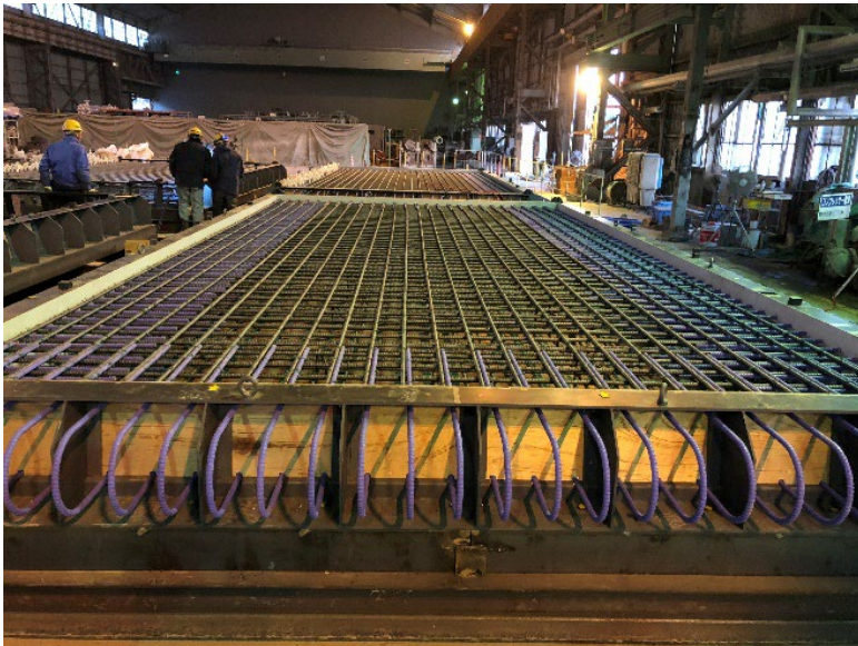
配筋の状況
