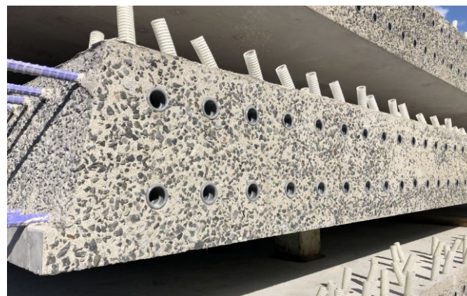
A部材の接合面
