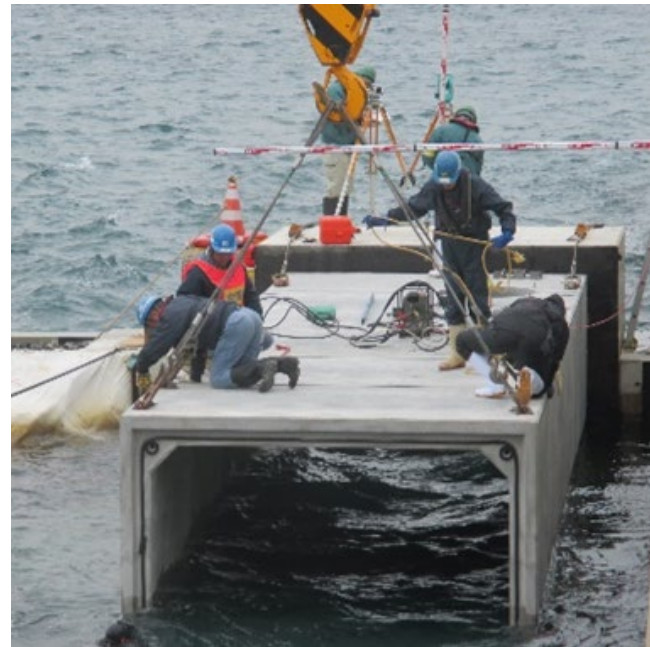
ボックスカルバート 九州地方整備局下関港湾事務所
