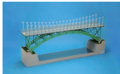
審査員特別賞 | 十網橋 秋田県立大館桂桜高等学校 土木・建築科 吉田 蓮 (3年) 鎌田 莞太 (3年) 橋本 さやか (3年) 渡辺 璃央 (3年)
